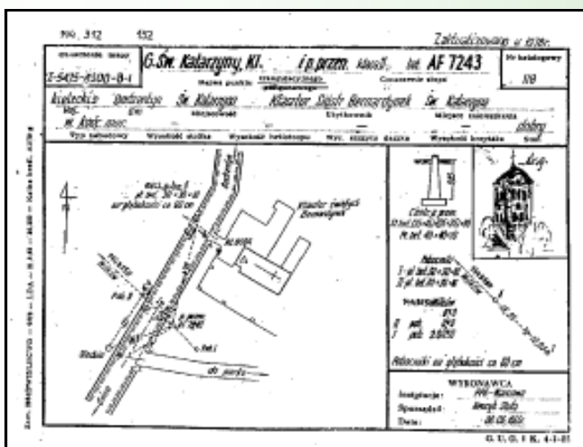
Opis topograficzny reperu początkowego
